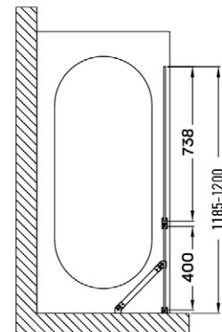
EDGE 120 BATHTUB PANEL
